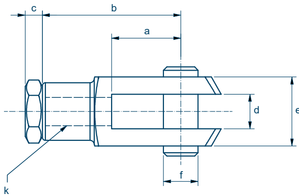
Gabelgelenk
