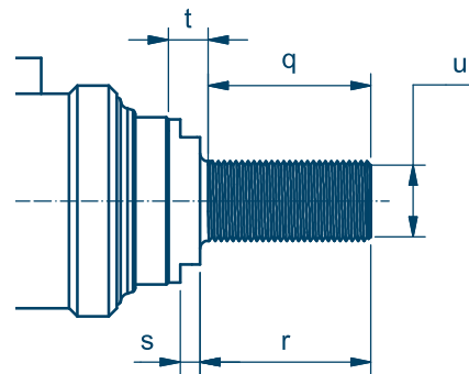
Außengewinde
